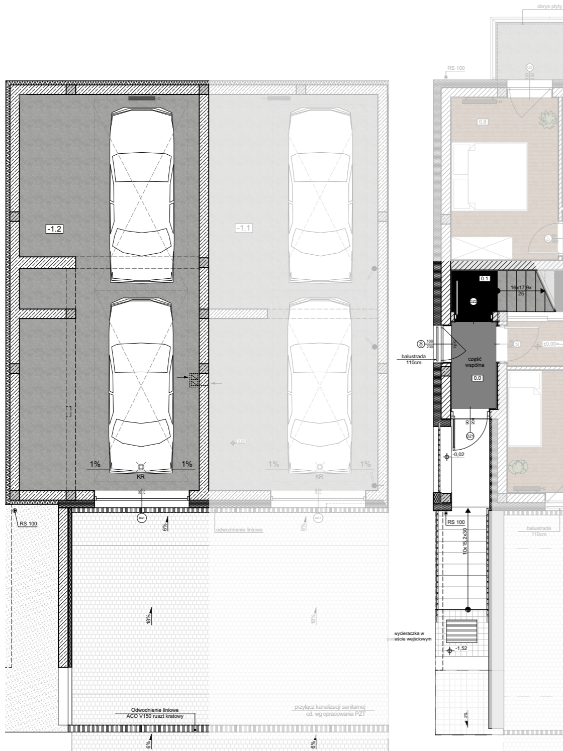
Rzut garażu indywidualnego -1
