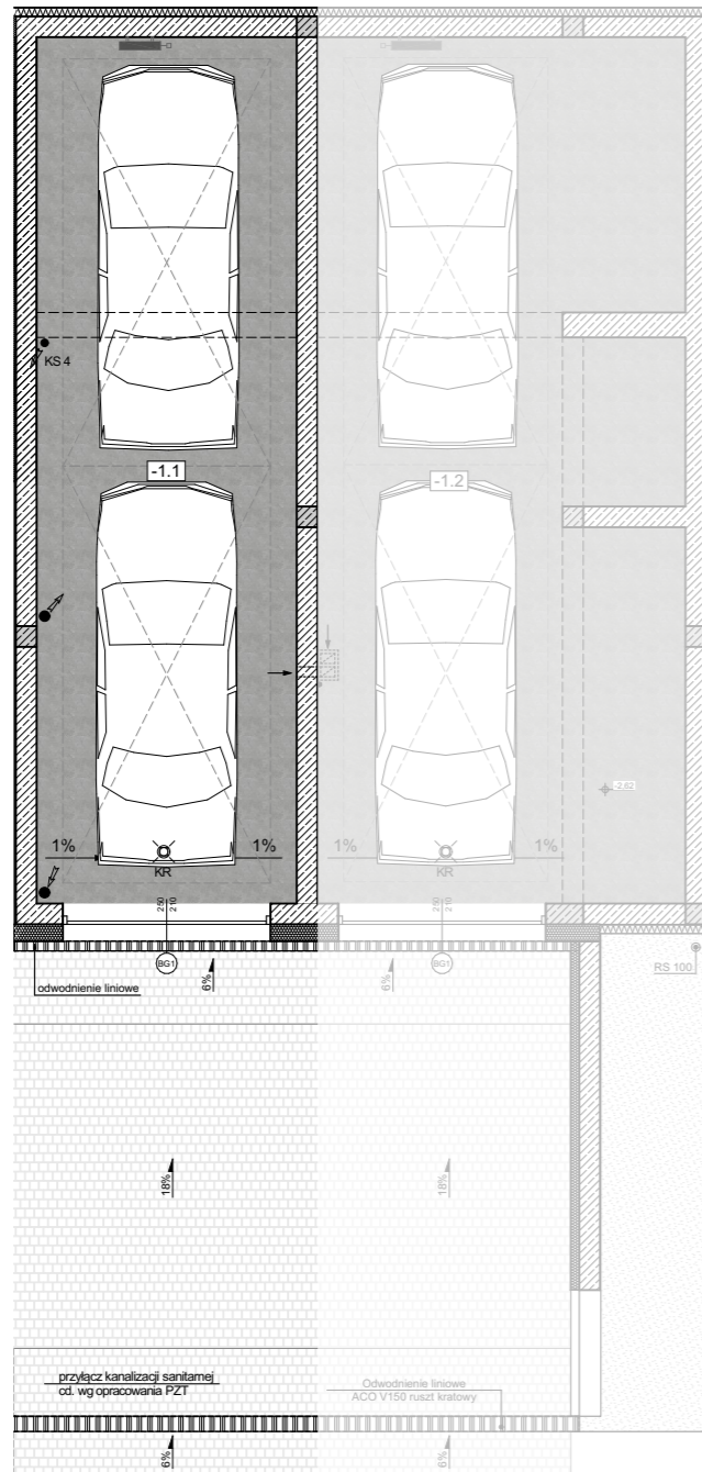
Rzut garażu indywidualnego -1
