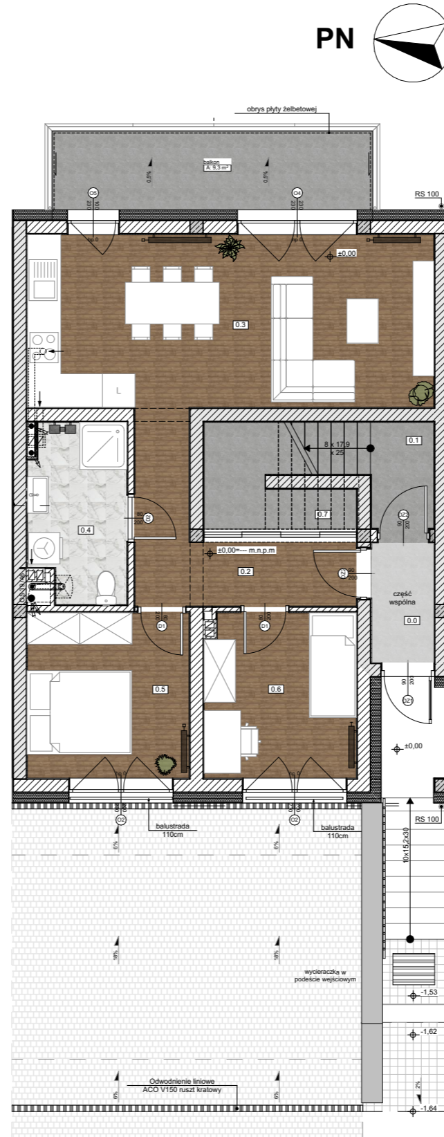
Rzut parteru 0
