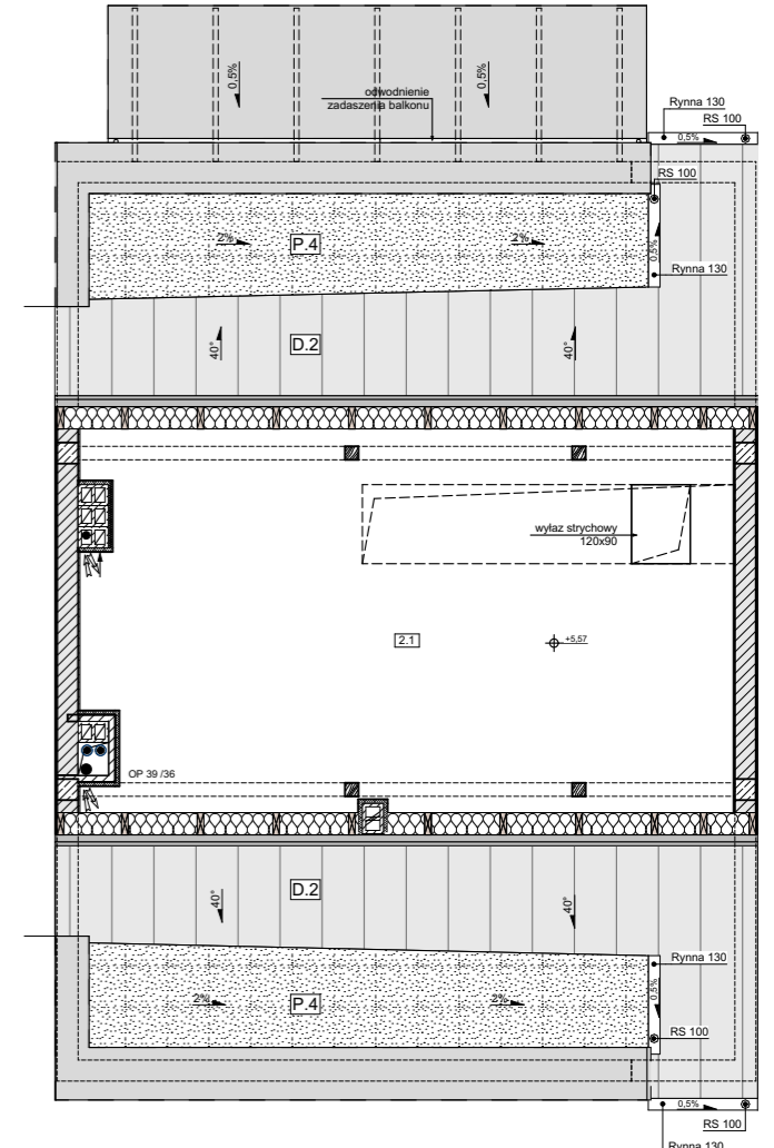
Strych +2
