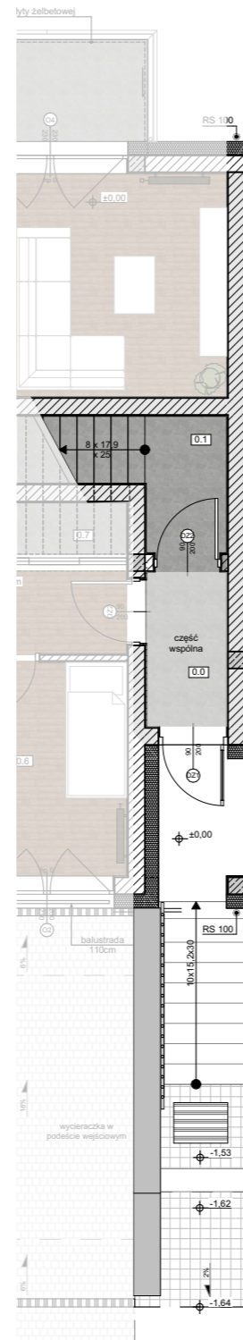
Rzut parteru 0
