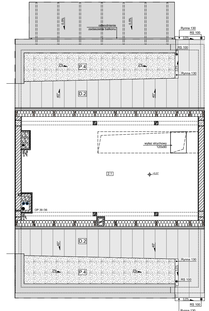
Strych +2
