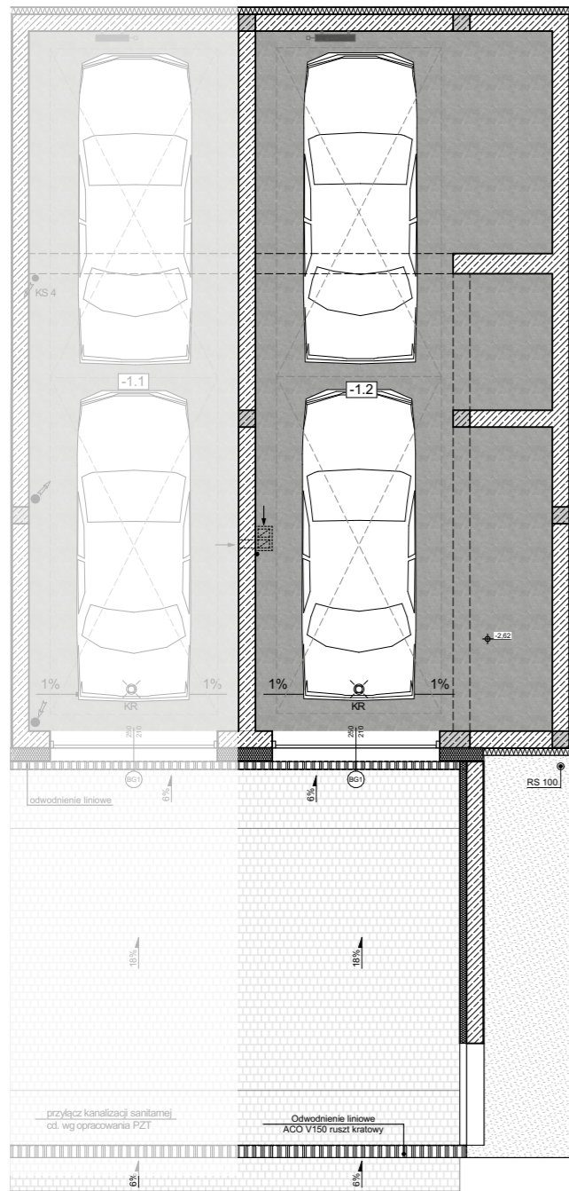
Rzut garażu indywidualnego -1
