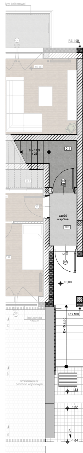
Rzut parteru 0
