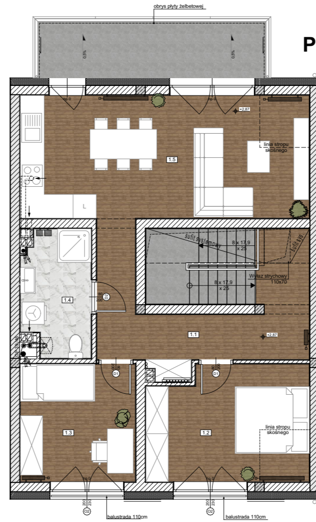
Rzut piętra +1
