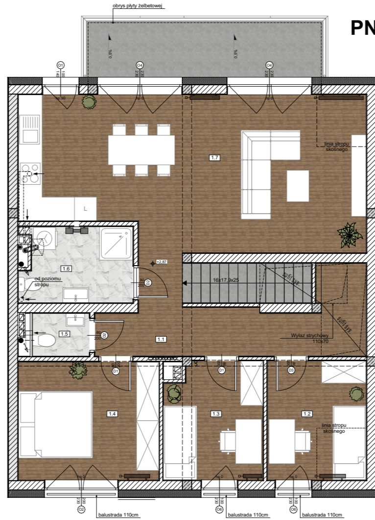
Rzut piętra +1
