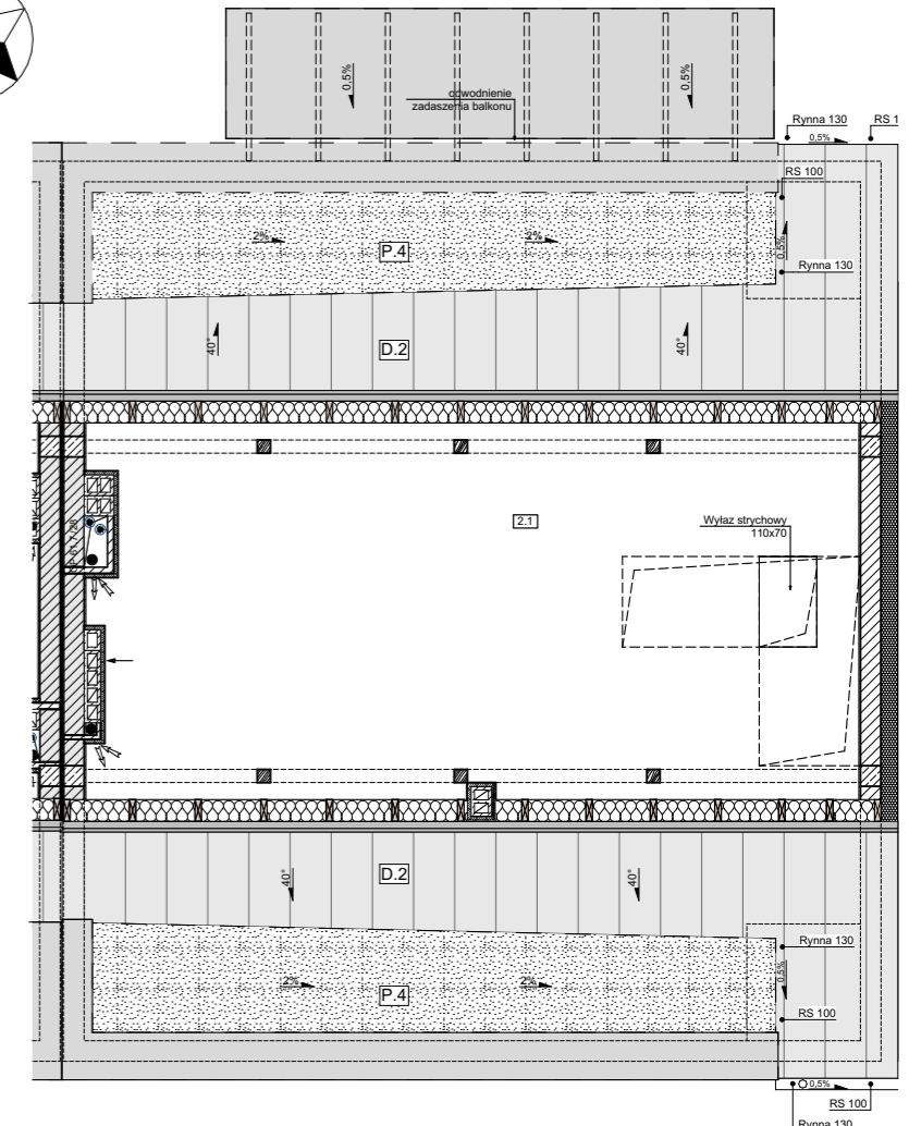
Strych +2
